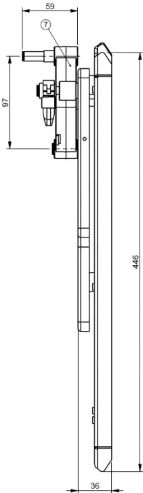
Fermator CSK-VF clutch assembly
